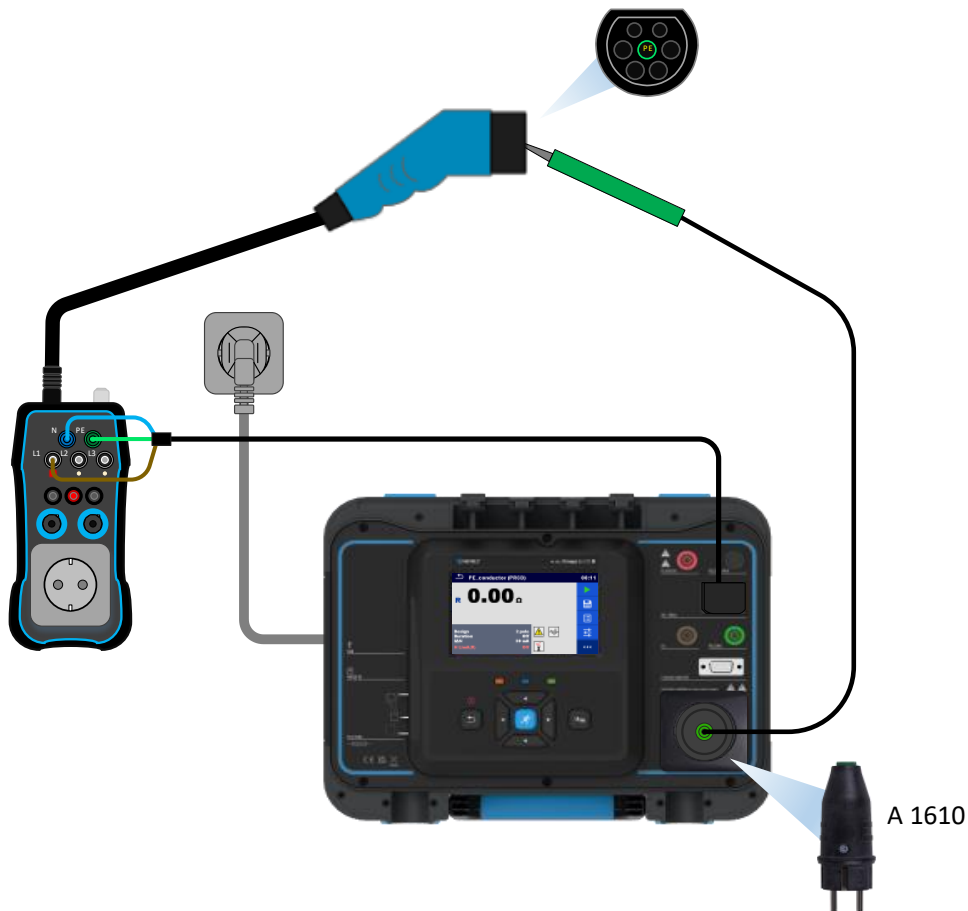
Abbildung 61_Kompensieren der Prüflleitungen
