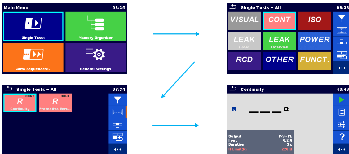
Abbildung 22_Aufbau der Widerstandsmessung
