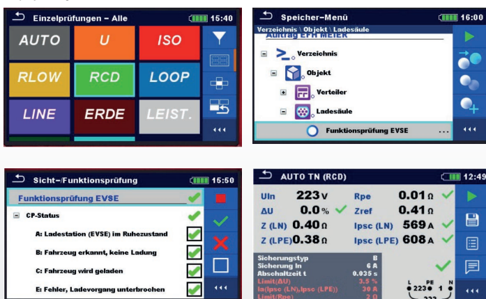
Displayanzeigen IT 200
