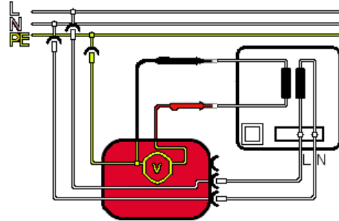
Stromlaufplan VDE 0544-4
