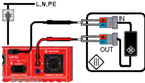
Anschlusschema VDE 0701-0702
