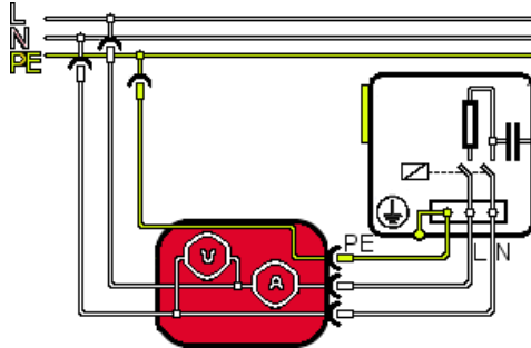
Stromlaufplan
