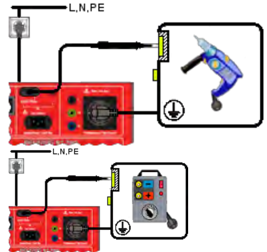
Anschlusschema VDE 0701-0702; VDE 0544-4
