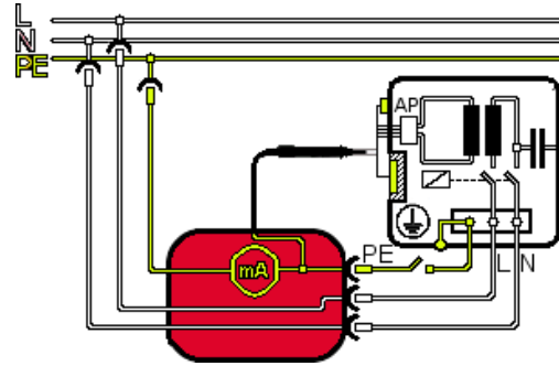
Stromlaufplan VDE 0751-1
