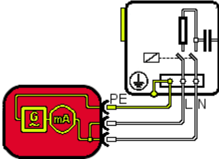
Stromlaufplan
