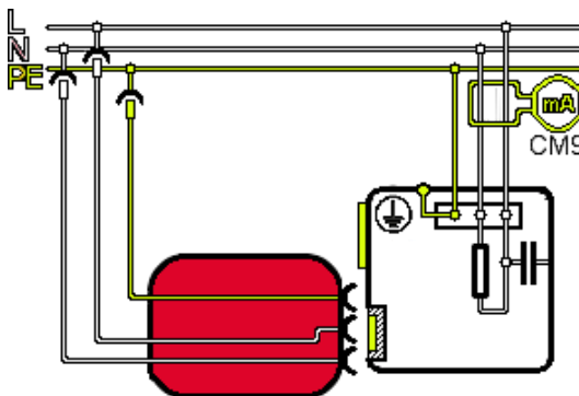
Stromlaufplan
