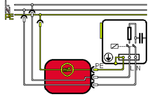
Stromlaufplan
