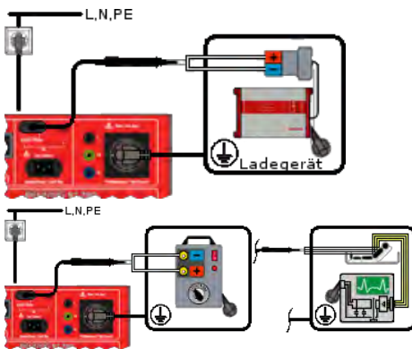
Anschlusschema
