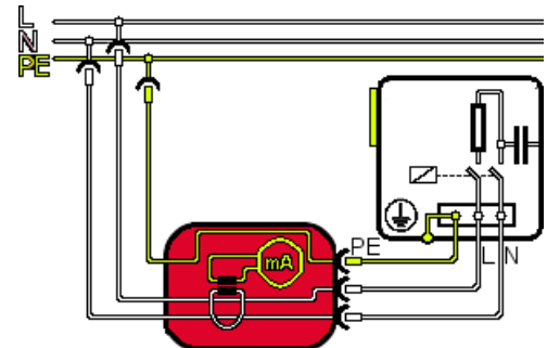
Stromlaufplan
