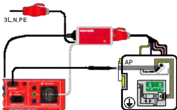
Anschlussschema VDE 0751-1
