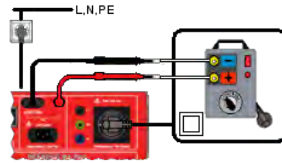
Anschlusschema VDE 0544-4
