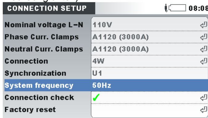
Abbildung 4.2: Menü Anschlusseinrichtung
