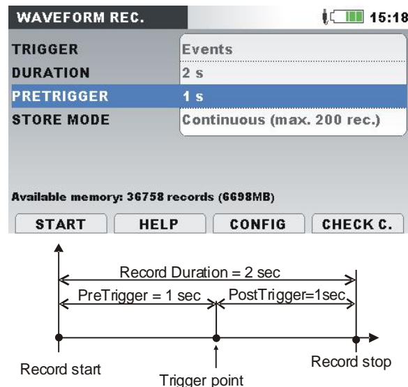
Abbildung 5.17: Darstellung der Auslösung und Vorauslösung
