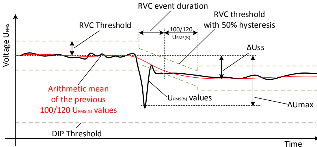
Abbildung 5.13: RVC Ereignisbeschreibung
