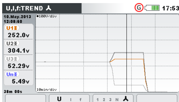
Abbildung 3.16: Spannungstrend (alle Spannungen)
