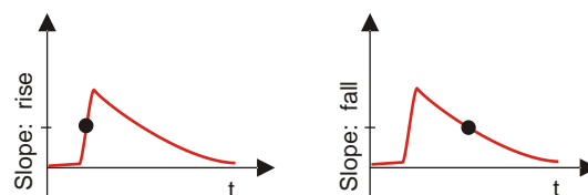
Abbildung 5.23: Flankenlösung
