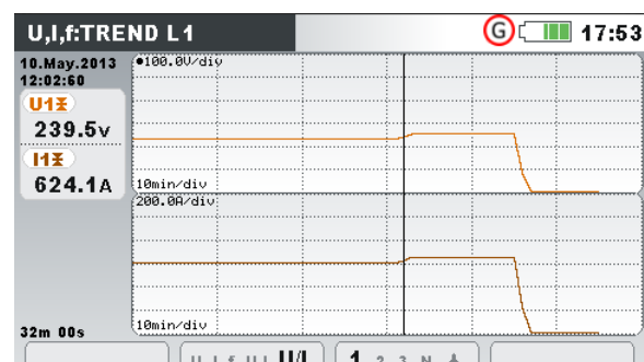
Abbildung 3.19: Spannungs- und
