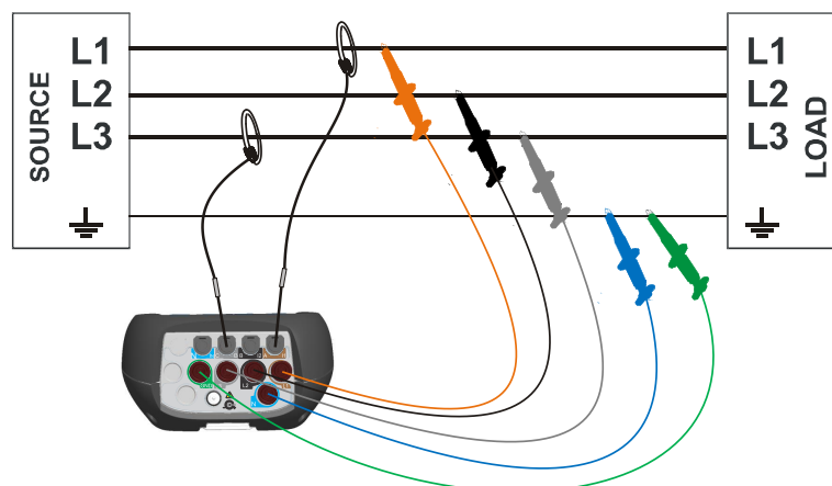
Abbildung 4.8: Offenes Dreieck-3-Leitersystem (Aaronschaltung)
