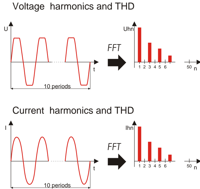
Abbildung 5.6: Strom- und Spannungsharmonische
