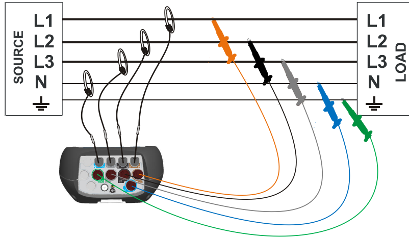
Abbildung 4.4: 3-Phasen 4-Leitersystem
