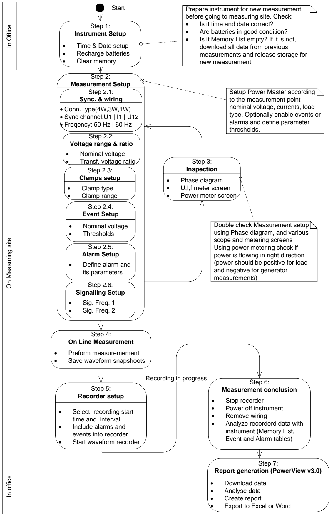
Abbildung 4.1: Empfohlenes Messverfahren
