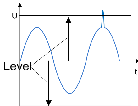
Abbildung 5.25: Feststellung des Transienten-Auslösers (Hüllkurve)
