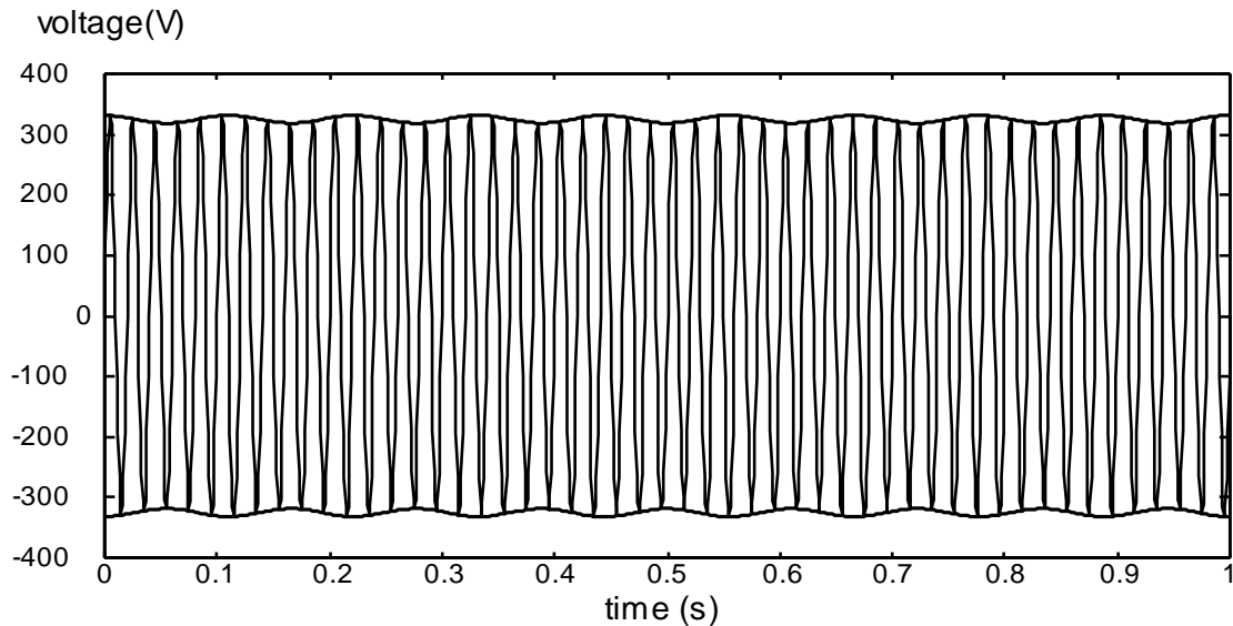
Abbildung 5.8: Spannungsschwankung
