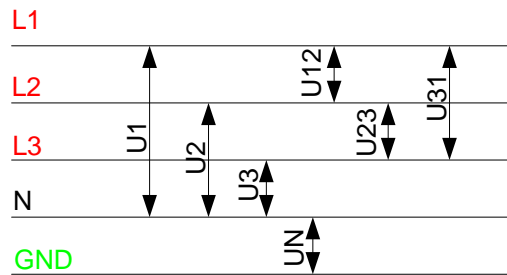
Abbildung 5.1: Phasen- und Phase-Phase-(Leiter)-Spannung
