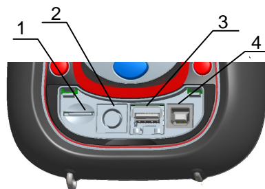
Abbildung 2.3: Seitliches Anschlussfeld
