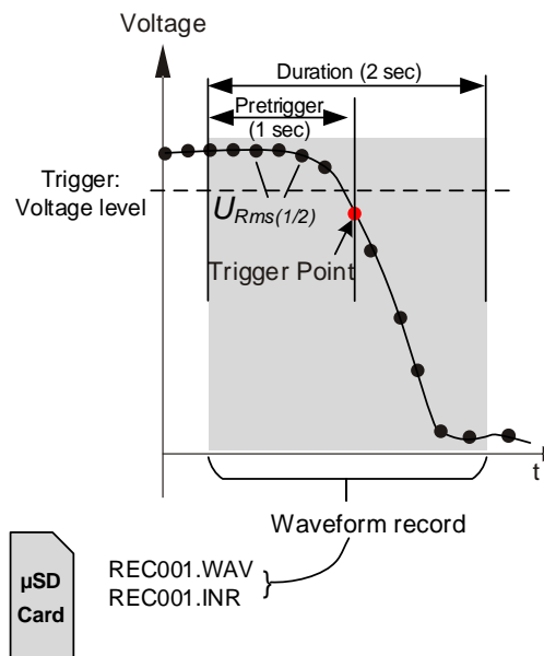
Abbildung 5.19: Spannungs-Niveau-Auslösung
