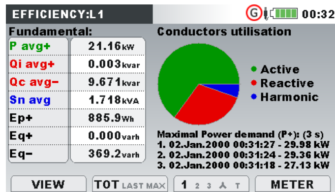
Abbildung 3.29: Bildschirm Energieeffizienz
