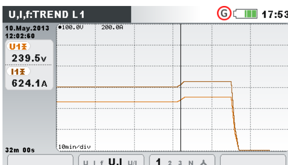
Abbildung 3.18: Spannungs- und
