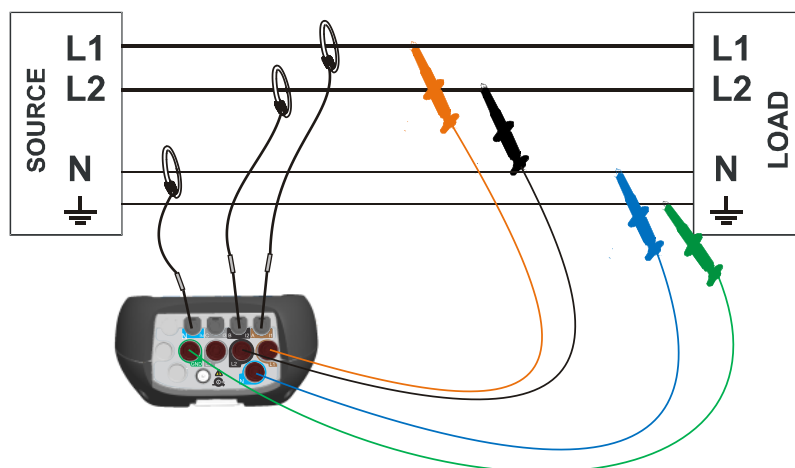
Abbildung 4.12: 2-Phasen 4-Leitersystem
