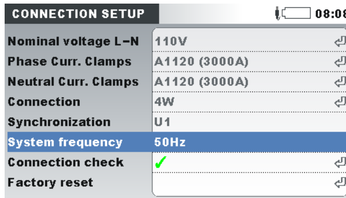
Abbildung 3.65: Bildschirm „ANSCHLUSSEINRICHTUNG
