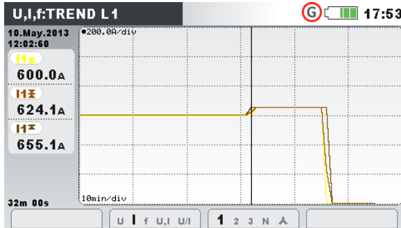
Abbildung 3.20: Trends aller Ströme
