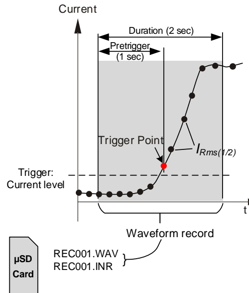
Abbildung 5.20: Strom-Niveau-Auslösung (Einschaltspitzen)
