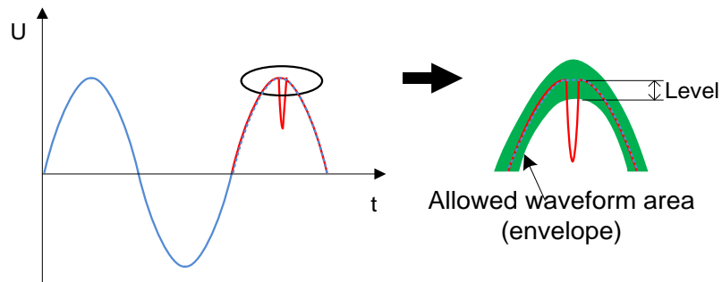
Abbildung 5.24: Feststellung des Transienten-Auslösers (Hüllkurve)
