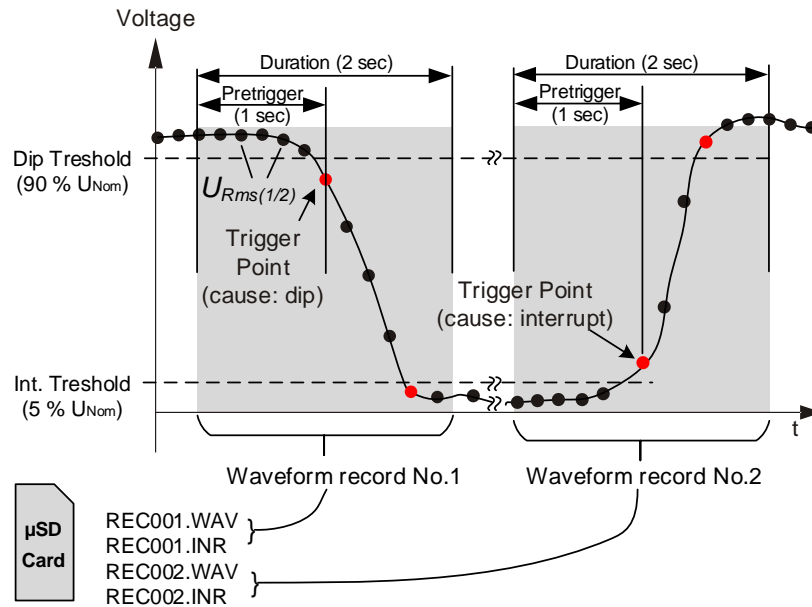
Abbildung 5.18: Spannungs-Ereignis-Auslösung
