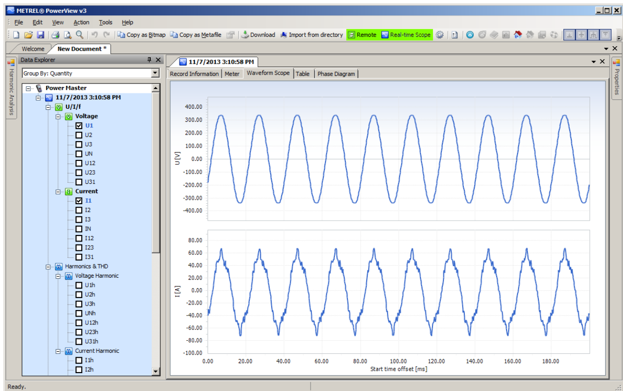
Abbildung 4.35: Fenster des Echtzeit-Oszilloskops bei einer Remote-Verbindung, mit verschiedenen, ausgewählten Kanälen
