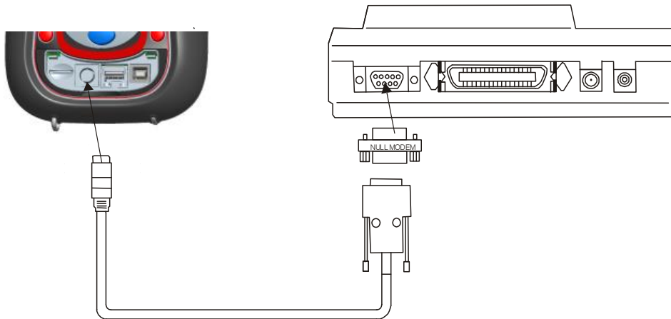
Abbildung 4.21: Anschließen des Druckers DPU 414 am Gerät
