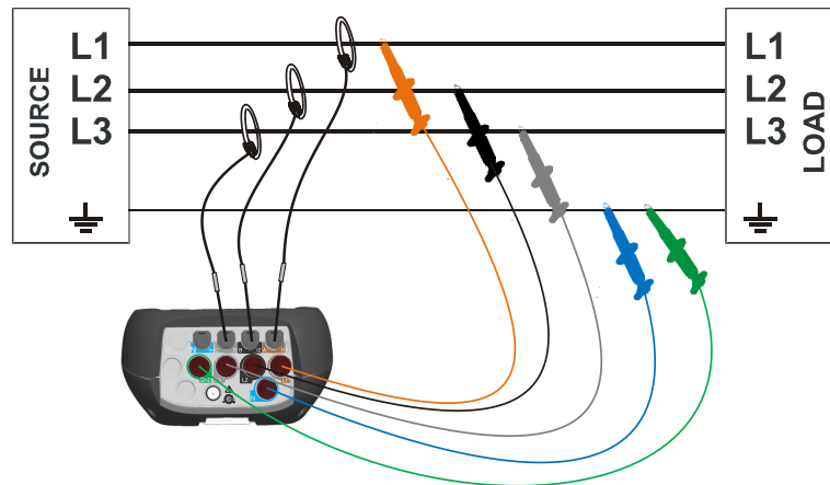
Abbildung 4.6: 3-Phasen 3-Leitersystem
